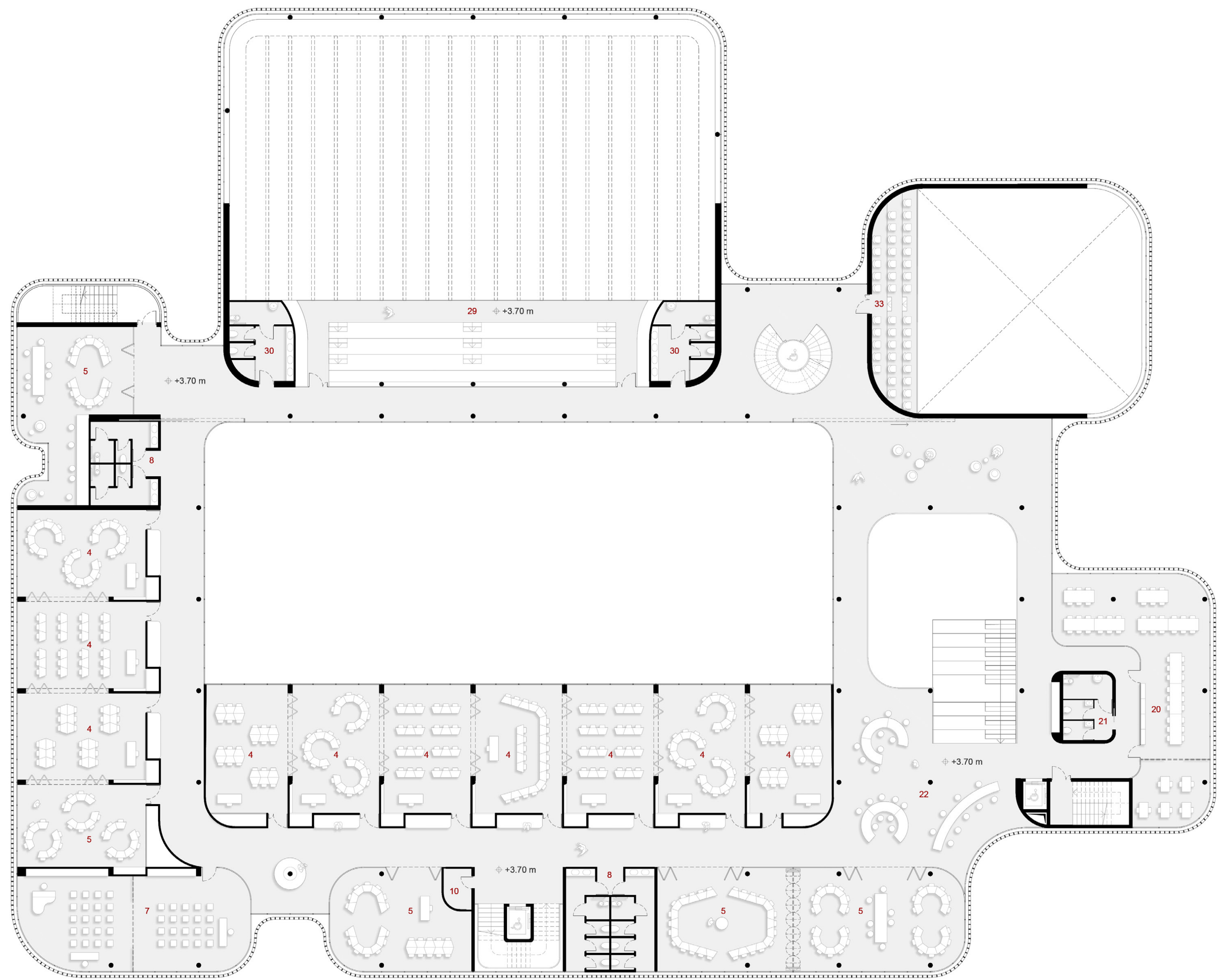
PIANTA PRIMO PIANO - 1:200
